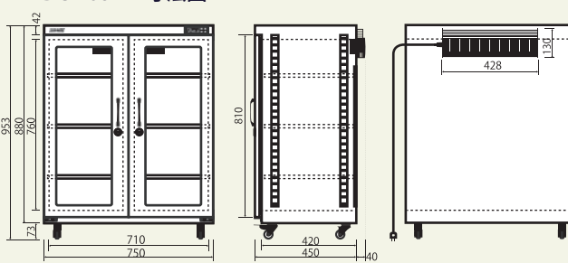
TDC-268-EX 寸法図
