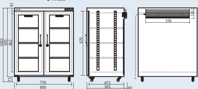
TDC-368-EX 寸法図
